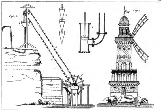
Machines hydrauliques.
