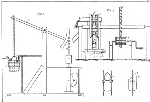
Machines hydrauliques.
