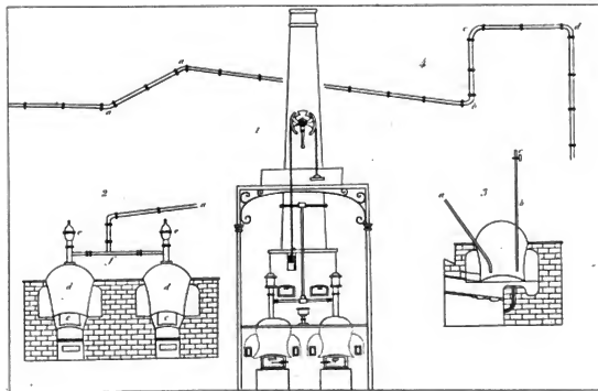
Machine à vapeur pour chauffer les Serres.
