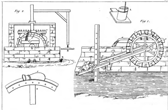
Machines hydrauliques.
