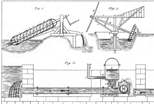
Machines hydrauliques.
