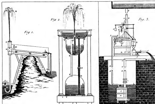
Machines hydrauliques.
