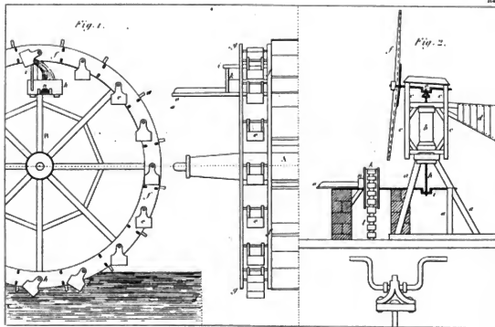
Machines hydrauliques.
